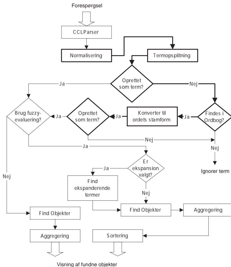
Figur 5.3: Flow-diagram over forespørgselsevalueringen, hvor de dele, der er sammenfaldende med behandlingen af objekter, er markeret.
